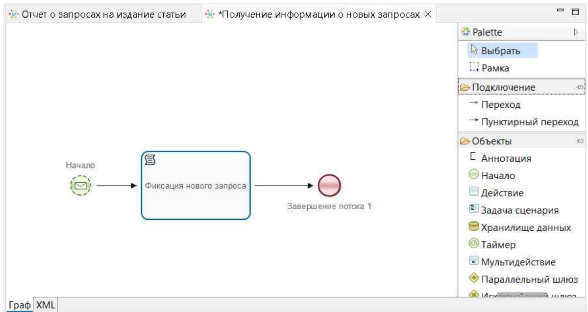
Рисунок 37. Вкладка «Граф» событийного подпроцесса
