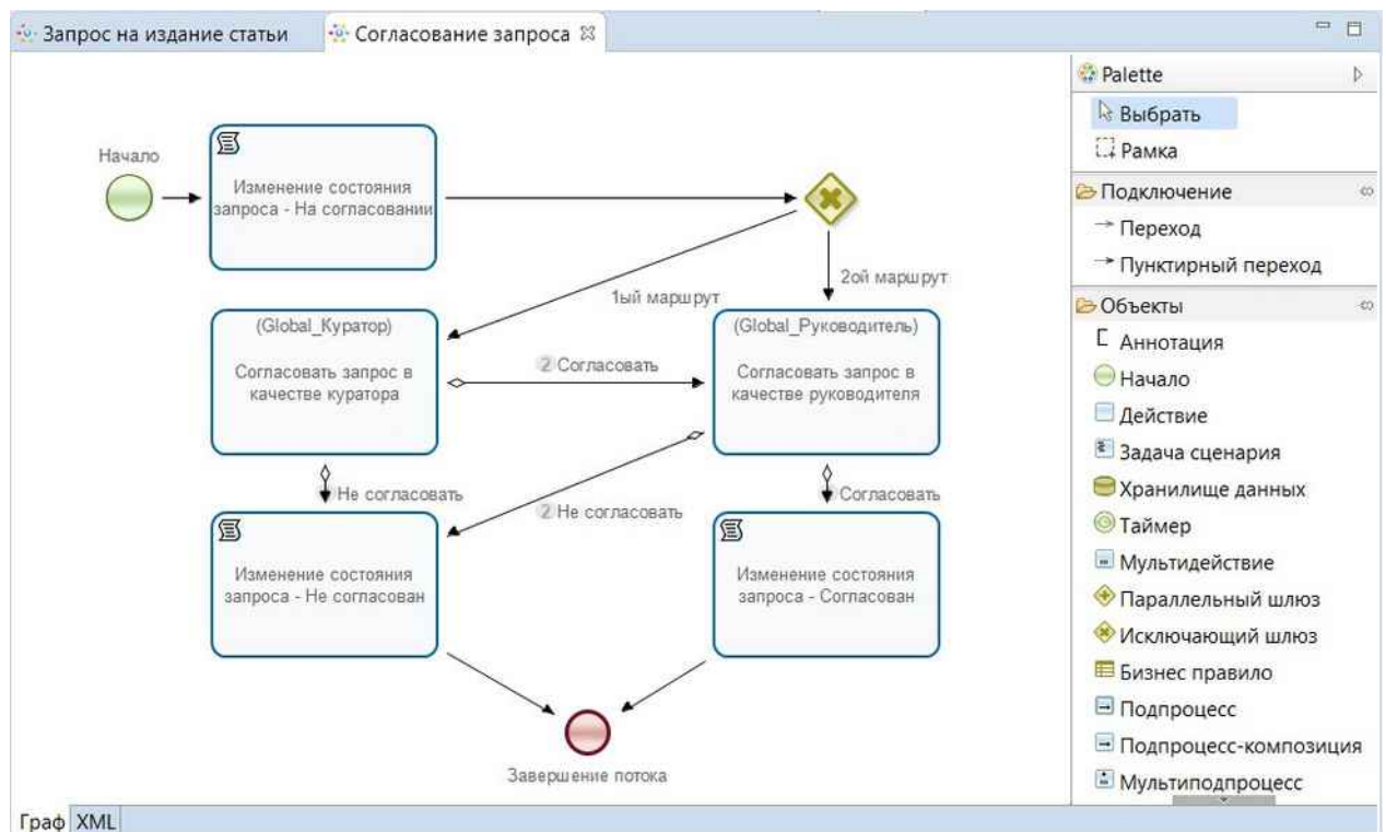
Рисунок 24. Вкладка «Граф» подпроцесса «Согласование запроса»
