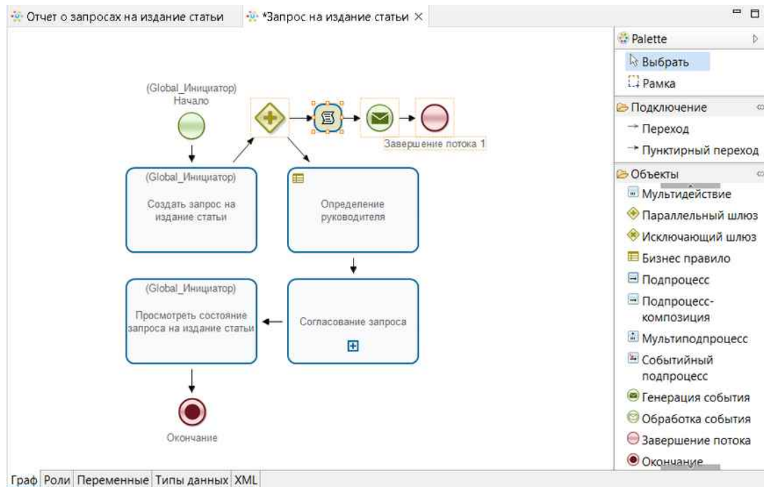
Рисунок 40. Добавление объектов в процесс «Запрос на издание статьи» (1)
