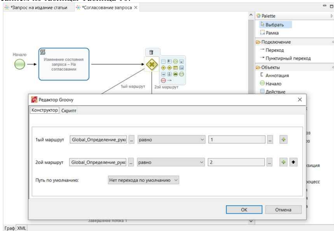
Рисунок 26. Конфигурация исключающего шлюза
