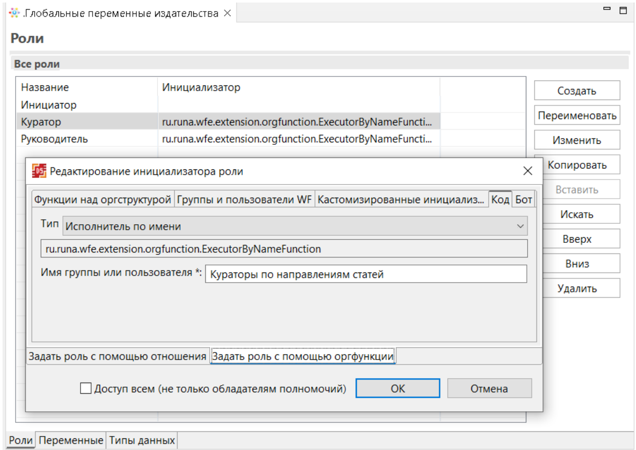
Рисунок 7. Инициализация роли «Куратор» по имени исполнителя
