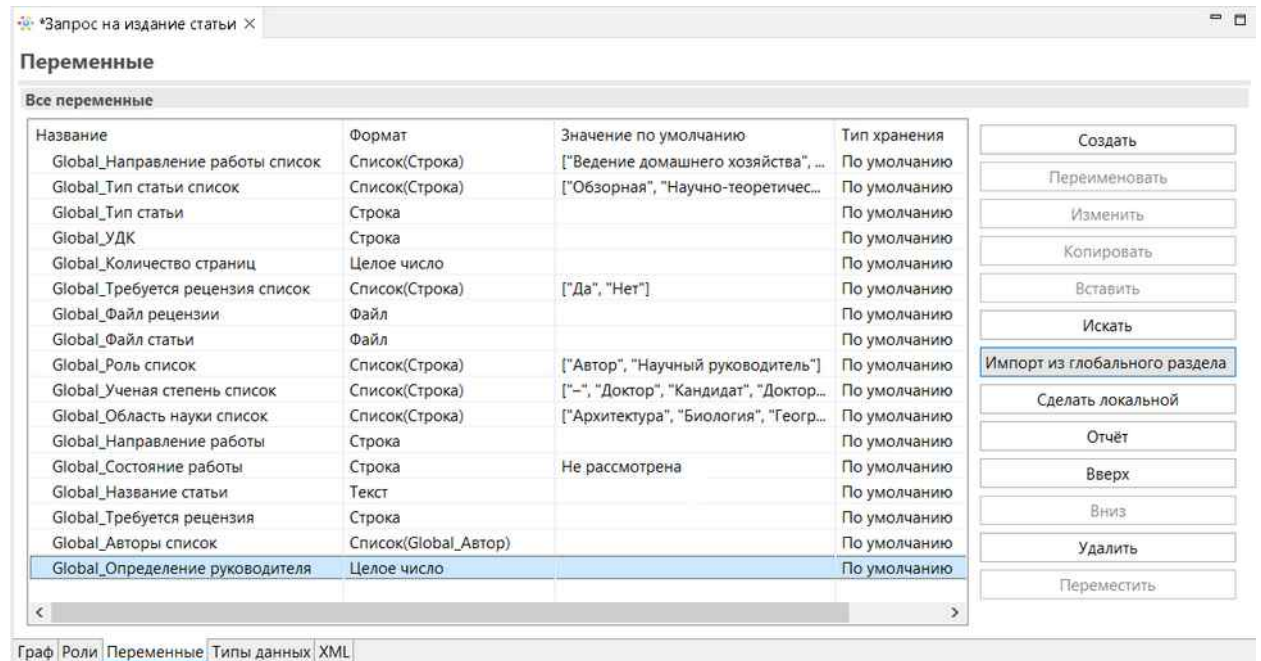
Рисунок 15. Вкладка «Переменные» процесса «Запрос на издание статьи» (1)
