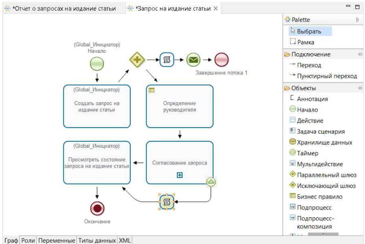
Рисунок 49. Добавление объектов в процесс «Запрос на издание статьи» (2)
