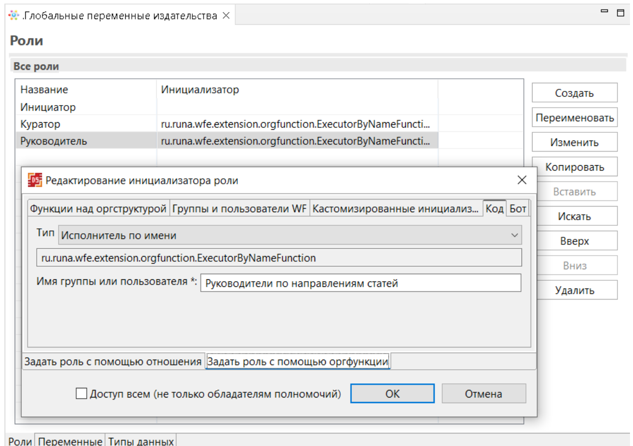
Рисунок 8. Инициализация роли «Руководитель» по имени исполнителя
