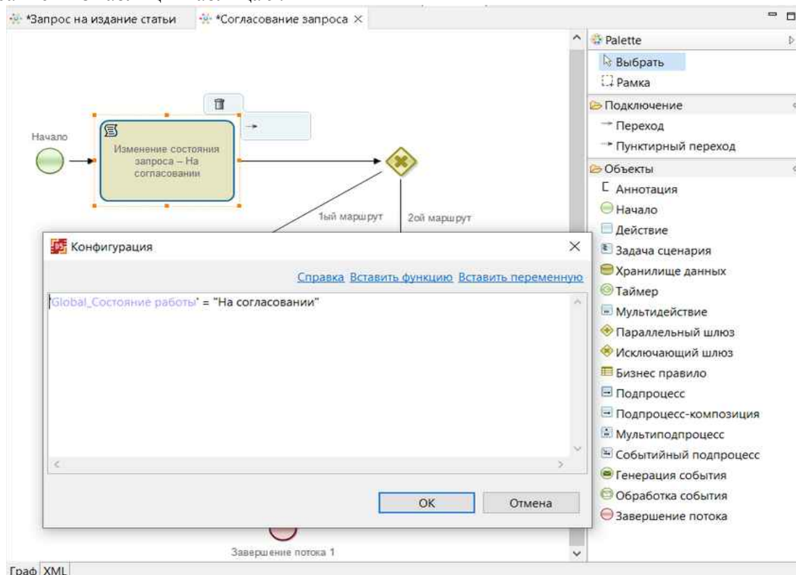
Рисунок 25. Конфигурация задачи сценария «Изменение состояния запроса – На согласовании»
