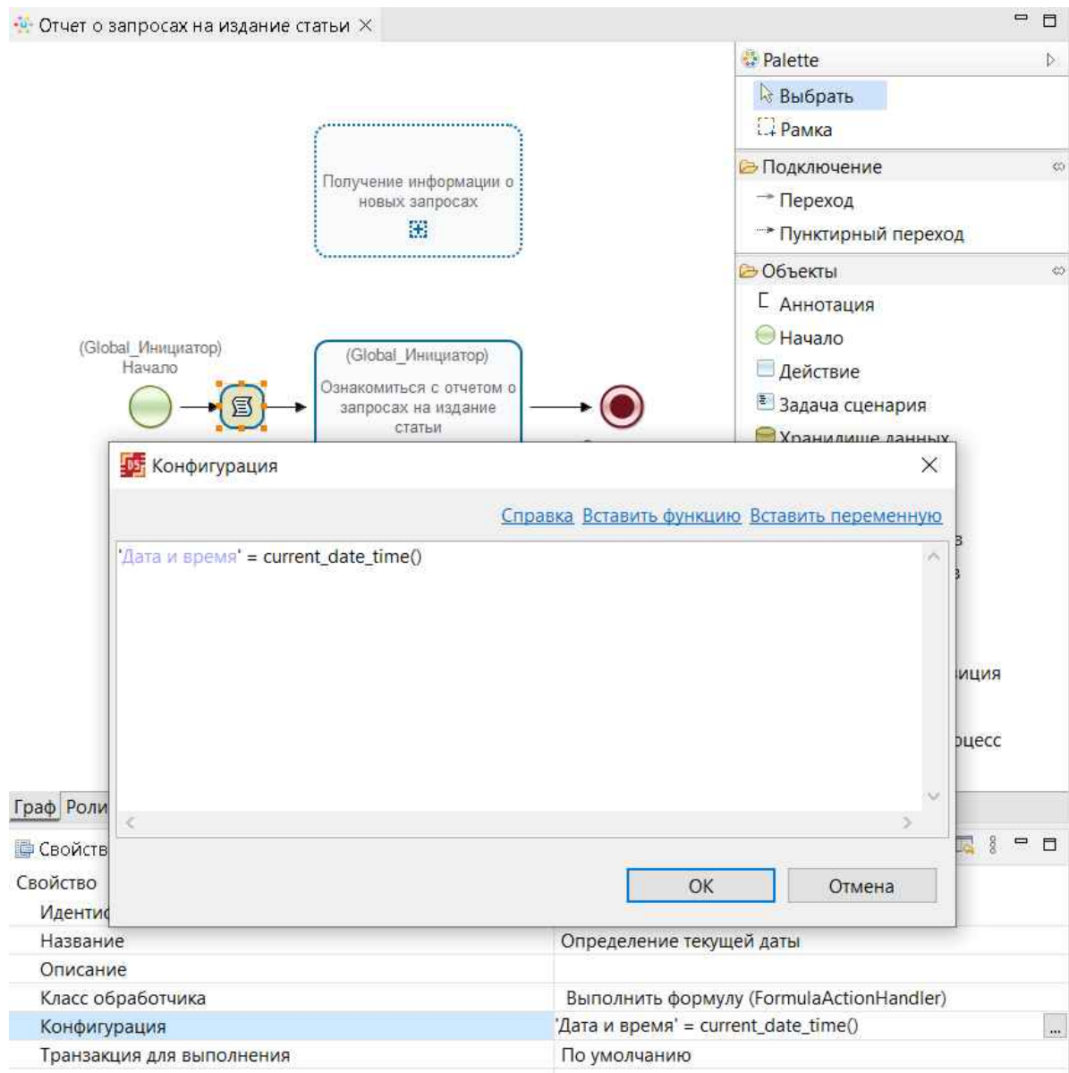
Рисунок 36. Конфигурация задачи сценария «Определение текущей даты»
