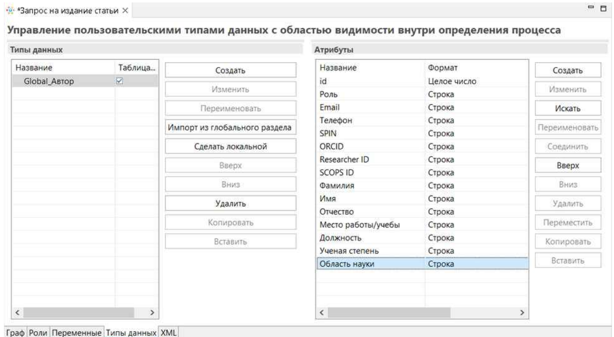
Рисунок 19. Вкладка «Типы данных» процесса «Запрос на издание статьи»
