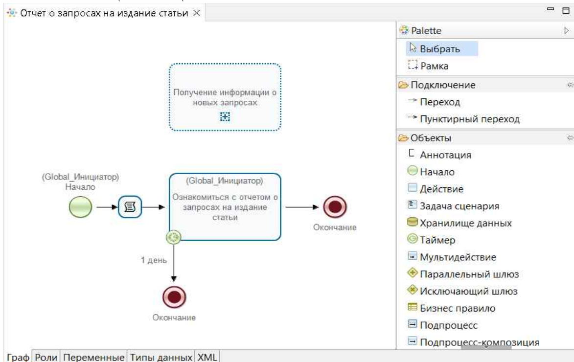
Рисунок 30. Вкладка «Граф» процесса «Отчет о запросах на издание статьи»
