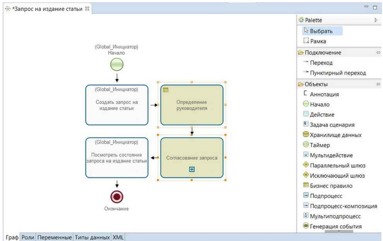
Рисунок 22. Добавление бизнес-правила и подпроцесса-композиции в процесс «Запрос на издание статьи»
